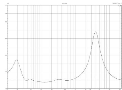
rys. 4. CE1TX , charakterystyka modułu impedancji.
